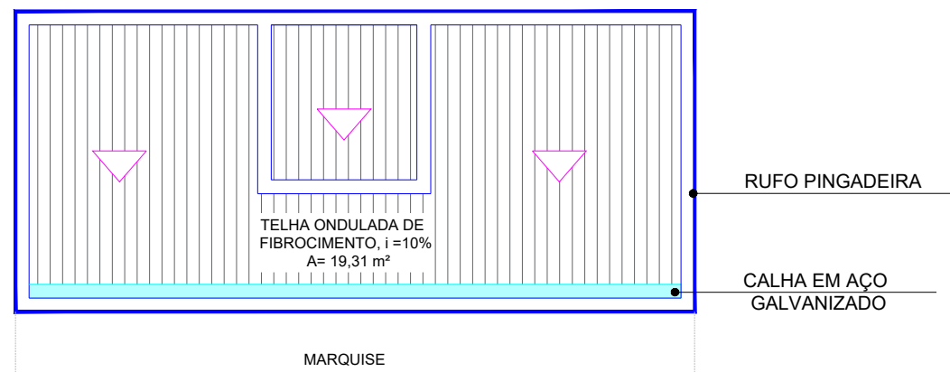
COBERTURA - TELHAMENTO E INCLINAÇÕES ESC. 1/75
