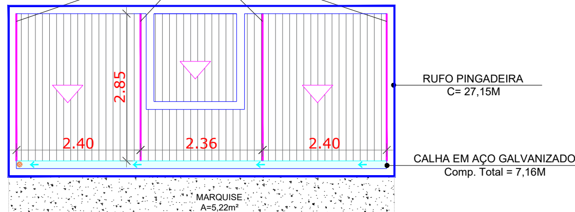
COBERTURA - DETALHES ESC. 1/75
