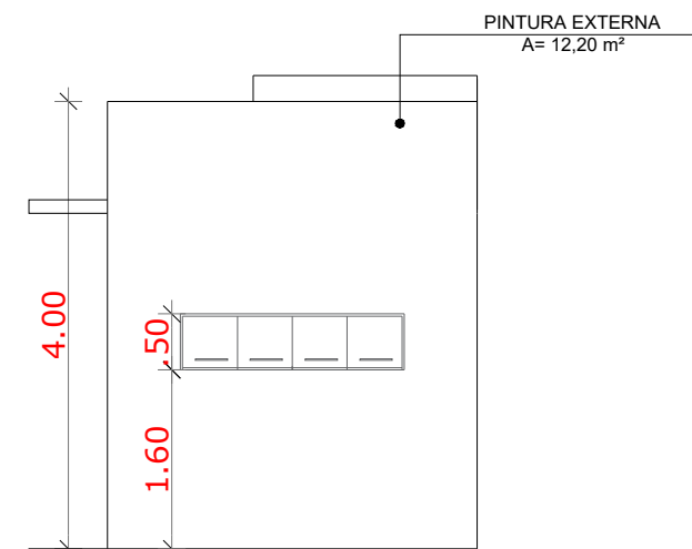
FACHADA LATERAL B ESC. 1/75
